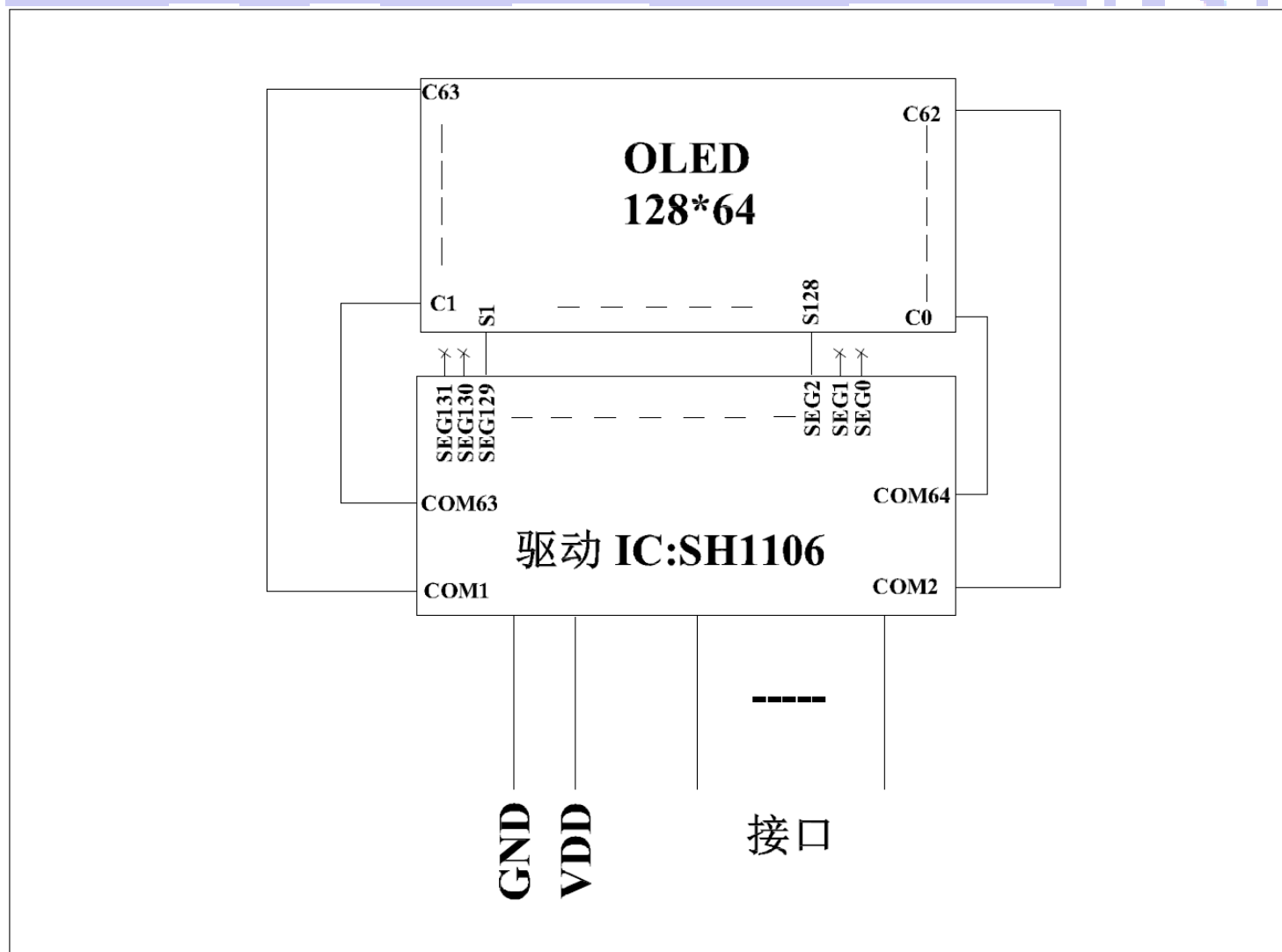
图 2: JLX12864OLED-13016-PC
