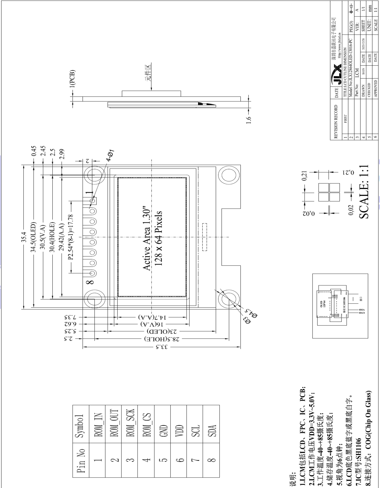
图 1. 外形尺寸
