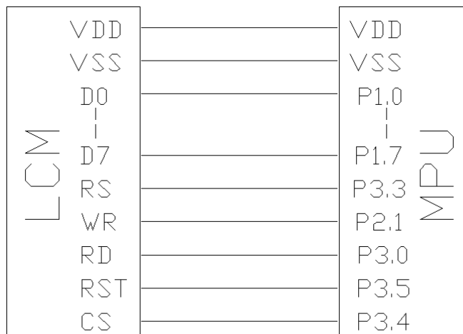
图 8: 并行接口图
