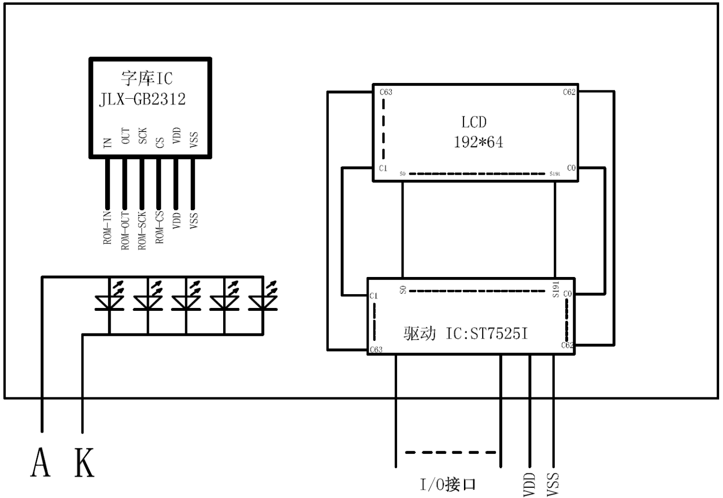
图 2: 电路框图
